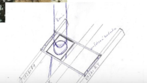
Stříkaná pěnová izolace Okolo nerezového svislého kouřovodu
